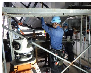
芯出し調整
