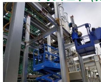
プッシャー架台 建て方
