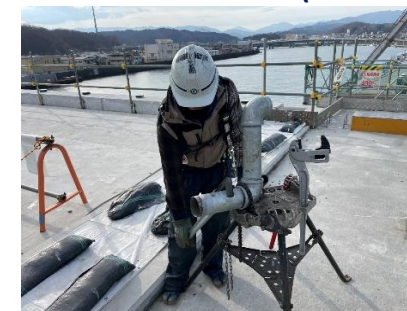
配管取外し解体中
